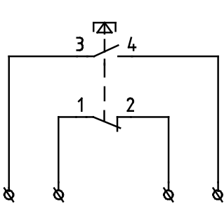
Left button
